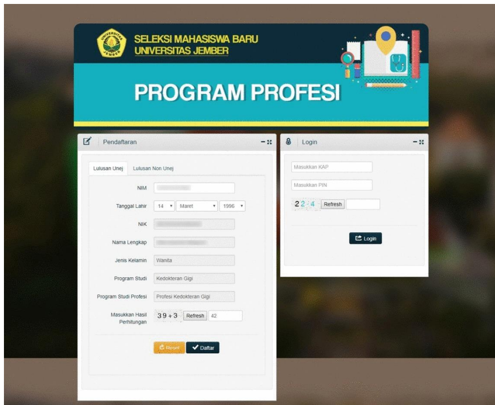
Gambar 2. Halaman Pendaftaran
